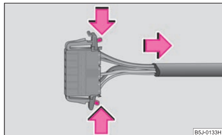
Obr. 192 Rozpojení svorkovnice
