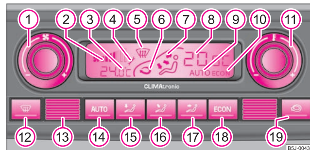
Obr. 97 Climatronic: ovládací prvky
