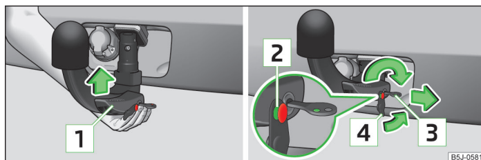
Obr. 107 Nasazení tažného ramena / zamknutí zámku a nasazení krytky zámku
