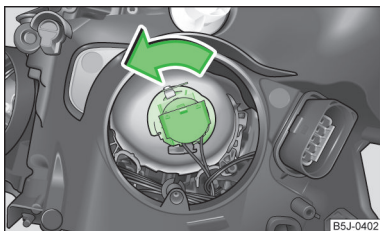
Obr. 158 Demontáž žárovky potkávacího světla
