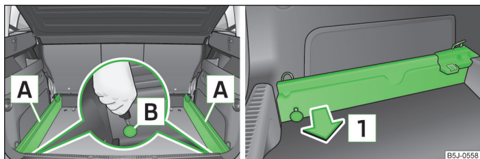
Obr. 52 Zavazadlový prostor: uvolnění pojistných bodů / vyjmutí nosných ližin
