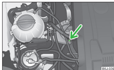
Obr. 149 Motorový prostor: kostřící bod
