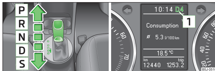
Obr. 93 Volicí páka / Informační displej: polohy volicí páky
