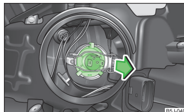
Obr. 157 Demontáž žárovky potkávacího a dálkového světla
