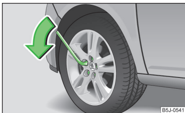
Obr. 143 Výměna kola: povelení šroubů
