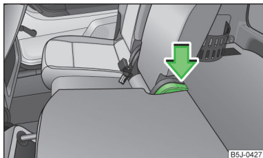
Obr. 44 Narovnání zádové opěry
