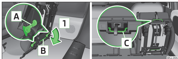
Obr. 42 Odjištění vyklopeného sedadla / Úchyty na sedáku
