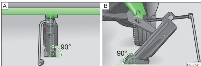
Obr. 145 Nasazení zvedáku vozidla
