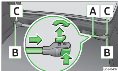
Obr. 54 Montáž příčniku
