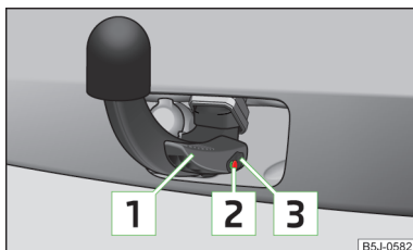
Obr. 108 Správné upnutí tažného ramena
