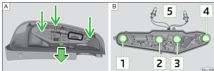
Obr. 165 Demontáž střední části svítilny / Rozmístění žárovek
