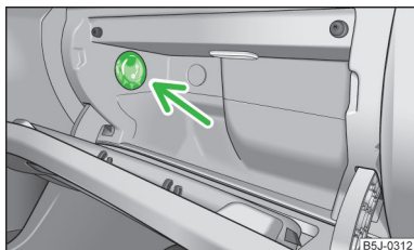
Obr. 64 Odkládací schránka: ovládání chlazení
