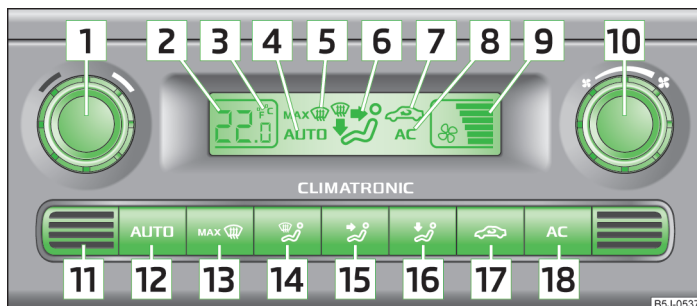
Obr. 84 Climatronic: ovládací prvky
