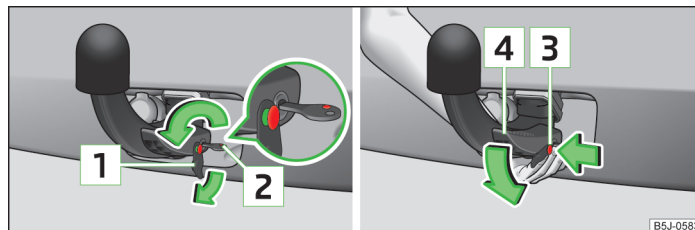
Obr. 109 Odemknutí ovládací páčky tažného ramena / uvolnění tažného ramena
