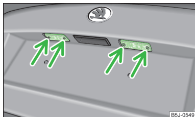
Obr. 163 Demontáž osvětlení registrační značky
