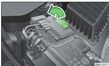
Obr. 133 Akumulátor: odklopení krytu
