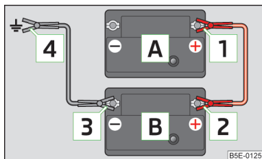
Obr. 148 Pomoc při startování: A - vybitý akumulátor, B - pomocný akumulátor
