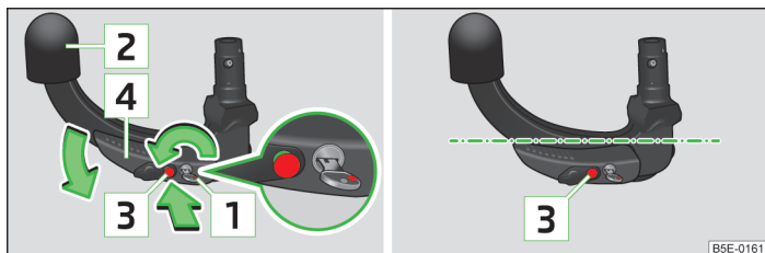
Obr. 106 Nastavení pohotovostní polohy / pohotovostní poloha
