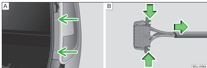
Obr. 164 Demontáž zadní skupinové svítilny / Rozpojení svorkovnice
