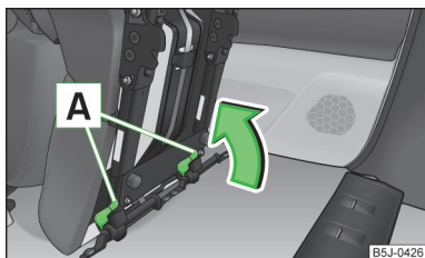
Obr. 43 Zajištění sedadla
