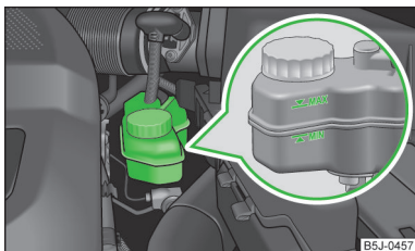
Obr. 132 Motorový prostor: nádržka brzdové kapaliny
