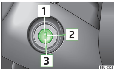
Obr. 105 Polohy klíče ve spínací skříňce
