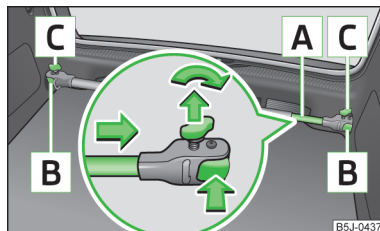
Obr. 70 Montáž příčnicku
