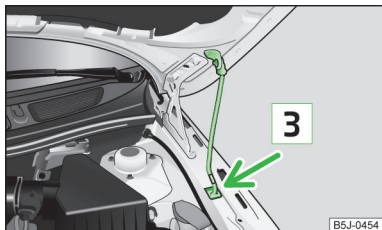
Obr. 128 Zajištění víka motorového prostoru
