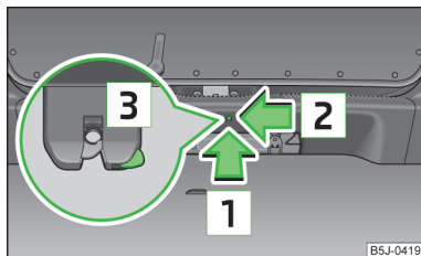
Obr. 36 Nouzové odemknutí víka zavazadlového prostoru
