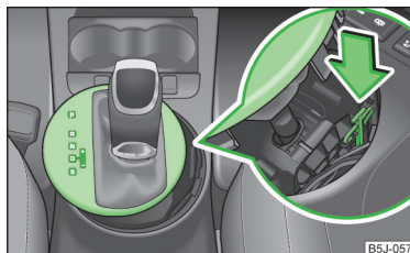
Obr. 110 Nouzové odblokování volič páky
