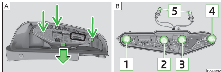
Obr. 166 Demontáž střední části svítilny / Rozmístění žárovek
