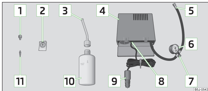
Obr. 148 Ilustrační obrázek: součásti sady na opravu pneumatik
