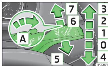
Obr. 48 Ovládací páčka: polohy ovládní stěračů a ostříkovačů skel
