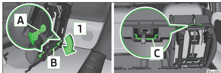
Obr. 57 Odjištění vyklopeného sedadla / Úchyty na sedáku
