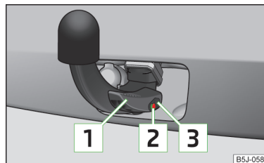
Obr. 124 Správné upnutí tažného ramena
