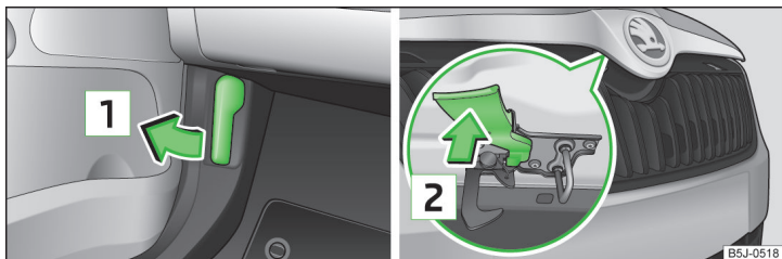
Obr. 127 Páčka pro odjištění víka motorového prostoru / páčka pojistky
