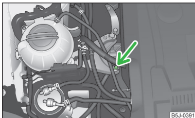
Obr. 150 Kostřící bod motoru: systém START-STOP
