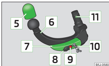
Obr. 121 Tažné rameno
