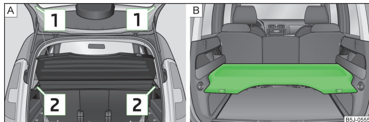
Obr. 64 Demontáž krytu zavazadlového prostoru / kryt zavazadlového prostoru v dolní poloze
