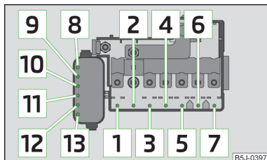
Obr. 156 Schematické zobrazení pojistek v motorovém prostoru
