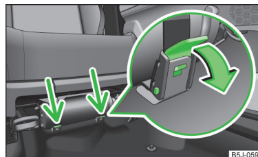
Obr. 142 Hasičí přístroj
