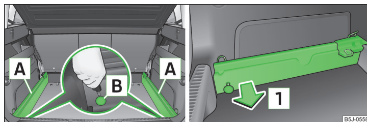
Obr. 68 Zavazadlový prostor: uvolnění pojistných bodů / vyjmutí nosných ližin
