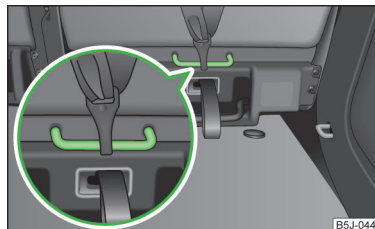
Obr. 17 Přichytné oko systému TOP TETHER
