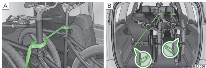
Obr. 73 Zajištění jízdních kol
