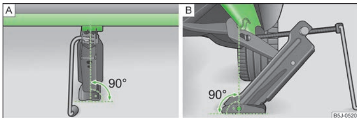
Obr. 132 Nasazení zvedáku vozidla
