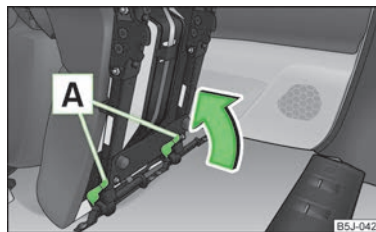
Obr. 42 Zajištění sedadla
