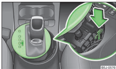
Obr. 88 Nouzové odblokování voliči páky
