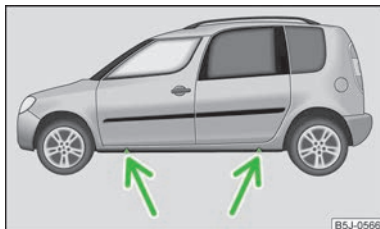
Obr. 131 Výměna kola: body pro nasazení zvedáku vozidla
