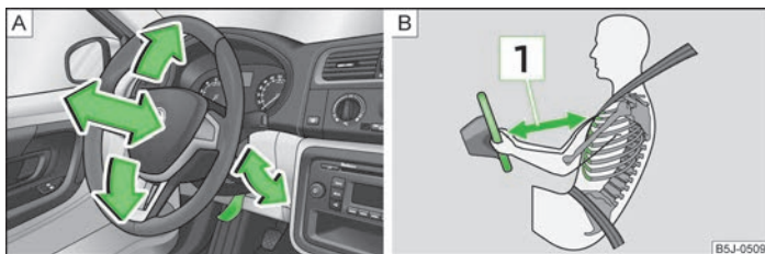
Obr. 78 Nastavitelný volant: páčka pod sloupkem řízení / Bezpečná vzdálenost od volantu
