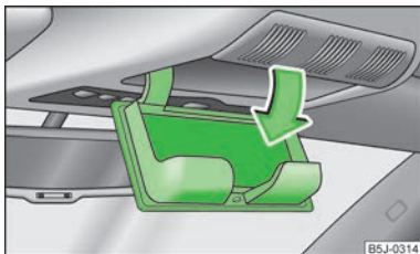
Obr. 65 Výřez ze stropního panelu: schránka na brýle
