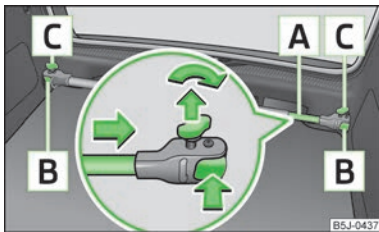
Obr. 53 Montáž příčnicku
