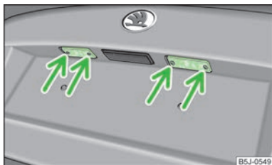
Obr. 150 Demontáž osvětlení registrační značky
