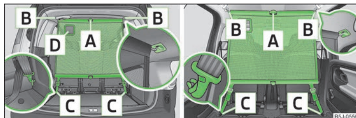
Obr. 48 Použití dělicí sítě za zadními / předními sedadly
