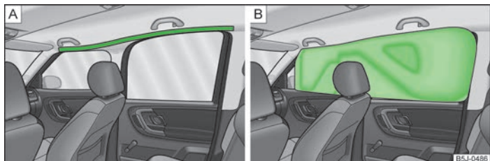
Obr. 102 Umístění hlavového airbagu / Hlavový airbag naplněný plynem
