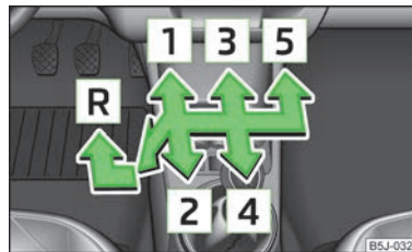
Obr. 82 Schéma řazení 5stupňové převodovky
